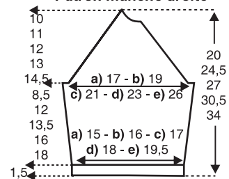
Patron manche droite
